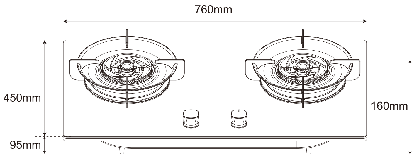
機身尺寸
