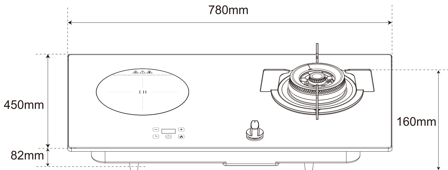
機身尺寸
